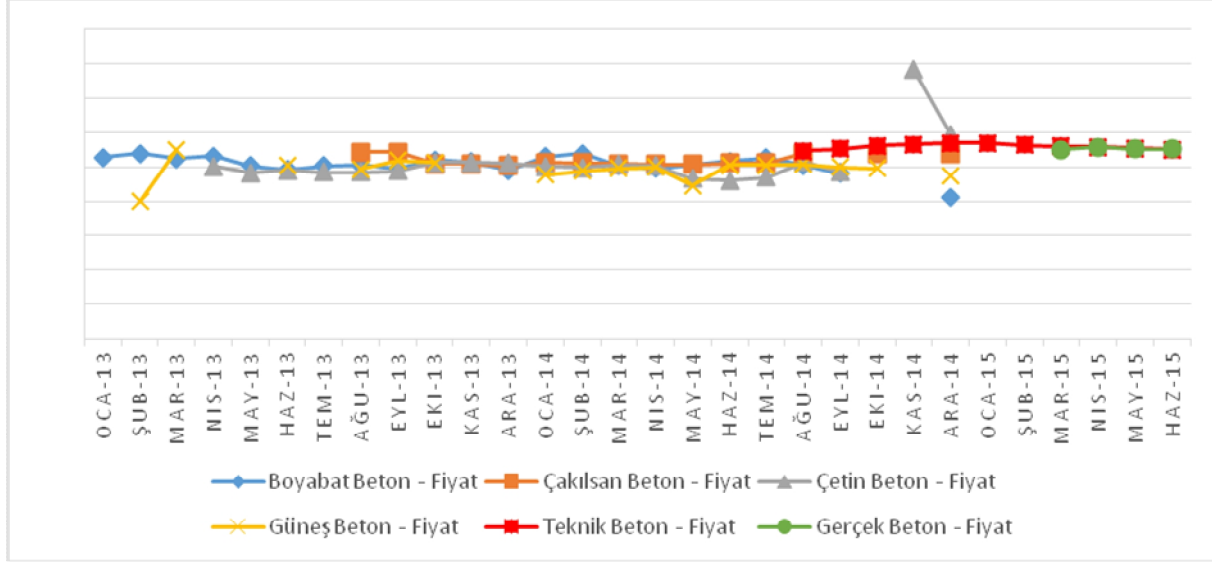
Grafik 1: Sinop Merkez Coğrafi Pazarı C25/30 Hazır Beton Türü Aylık Ağırlıklı Ortalama Fiyatları (TL/m 3 )
