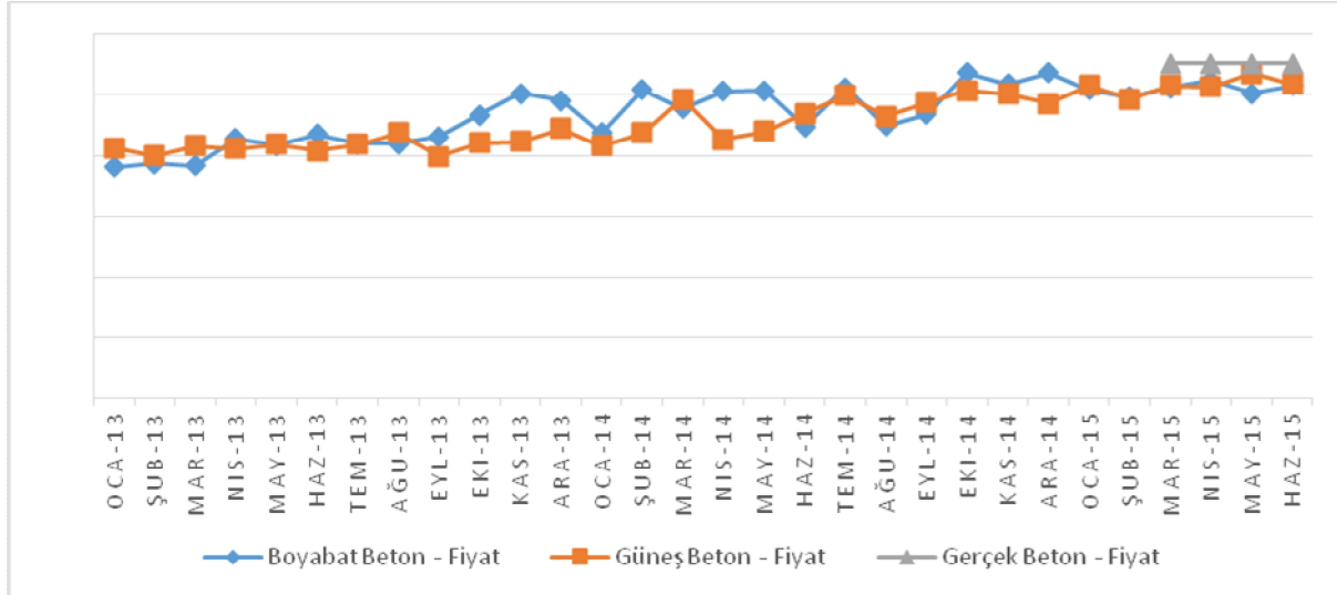
Grafik 3: Boyabat Coğrafi Pazarı C25/30 Aylık Ağırlıklı Ortalama Fiyatları (TL/ m 3 )
